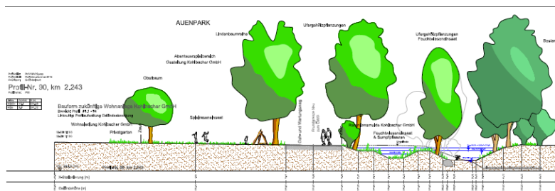
Landschaftsökologische Fachplanung Hochwasserschutz Schöckelbach, 3. Bauabschnitt, Graz, Bauformen
