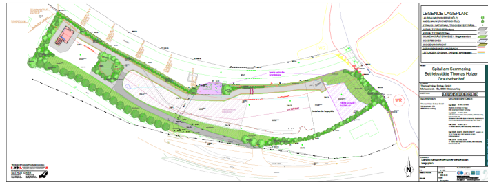
Bestandssituation mit Semmeringbahn & Landschaftspflegerischer Begleitplan Betriebsstätte Grautschenhof
