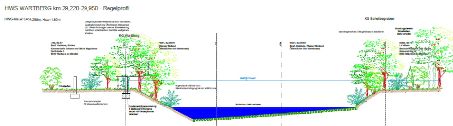
Ökologische Begleitplanung, Schnitt Hochwasserschutz Mürz, Gemeinde St. Barbara
